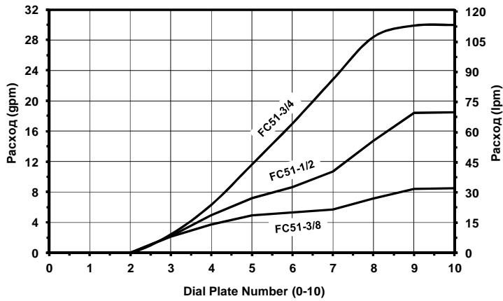
Величина расхода по шкале FC Series
