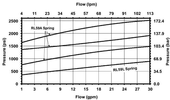
Зависимость давления от расхода FCR51
