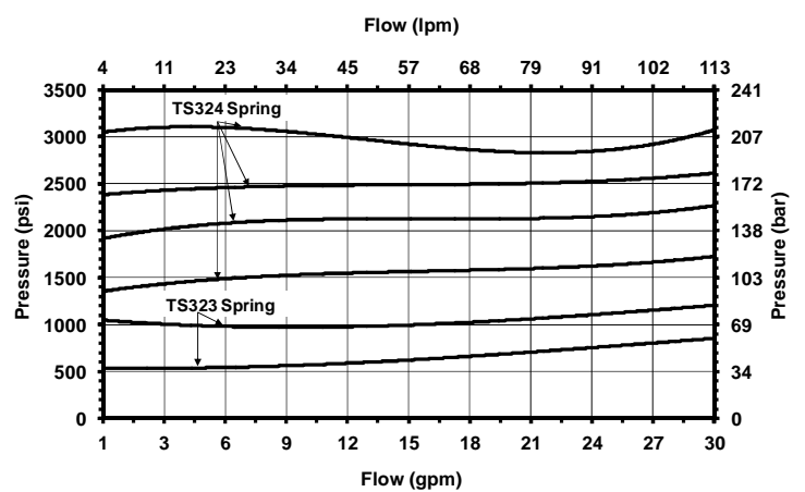
Зависимость давления от расхода FCB51
