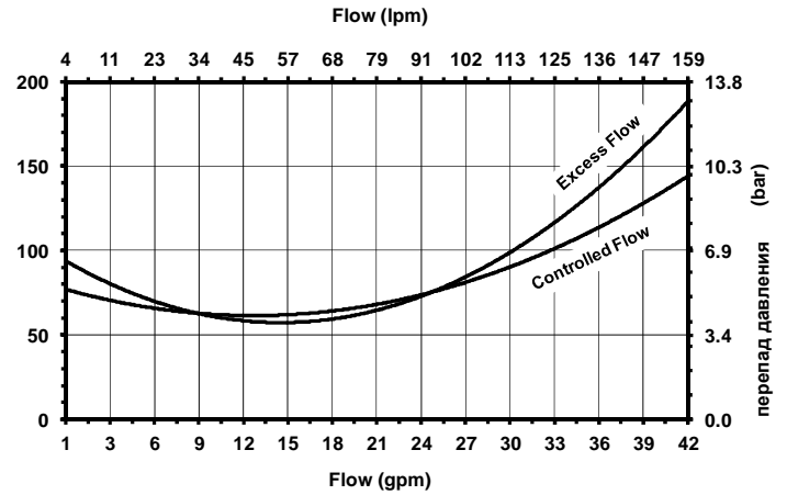
Перепад давления FC Series
